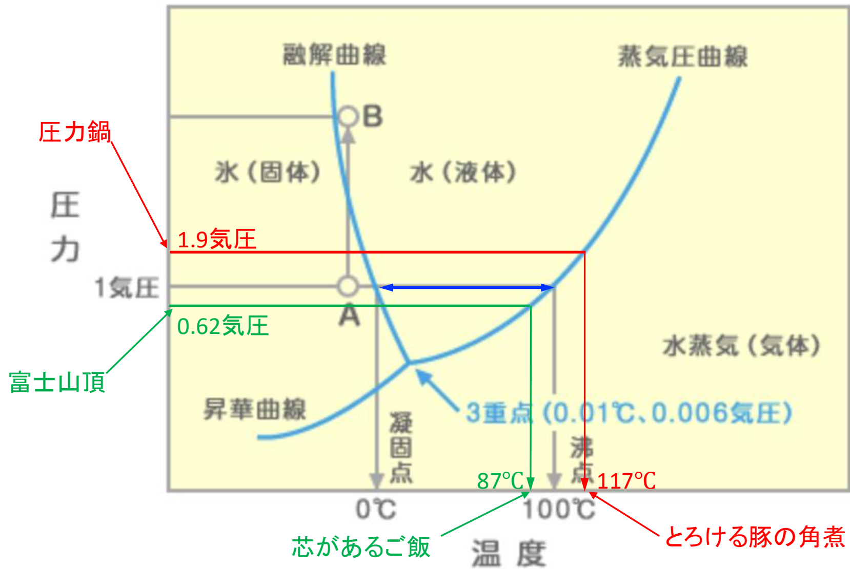
水の三相図
