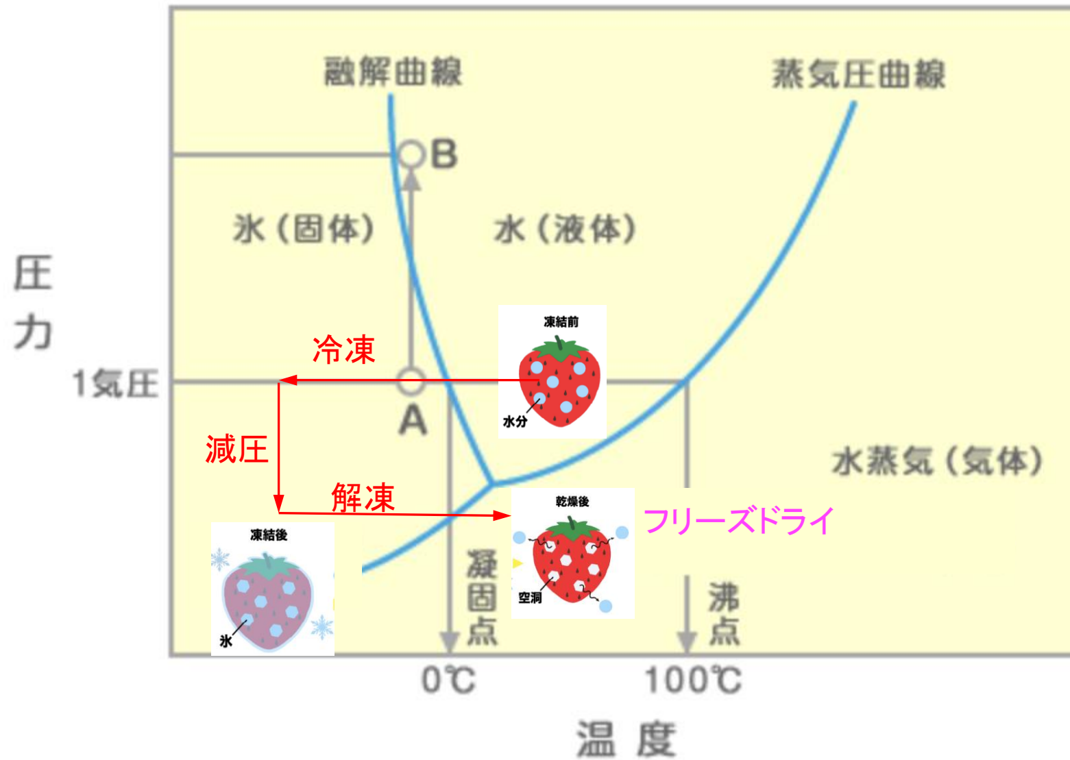
水の三相図
