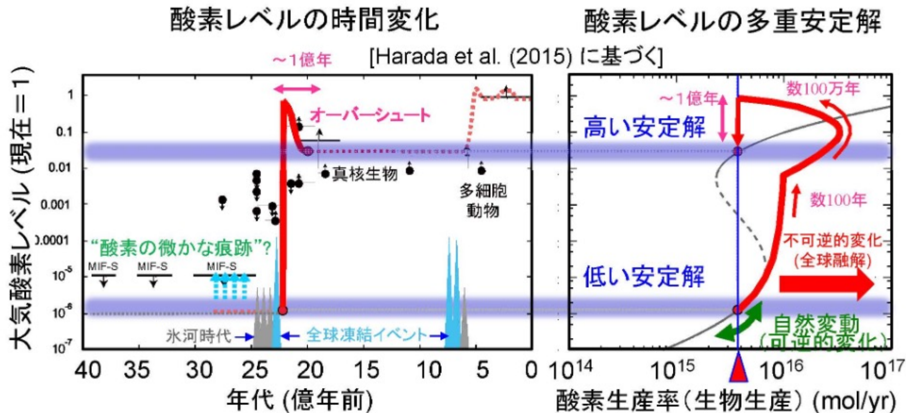
図6: 酸素濃度の安定レベルの遷移 (計算結果)
