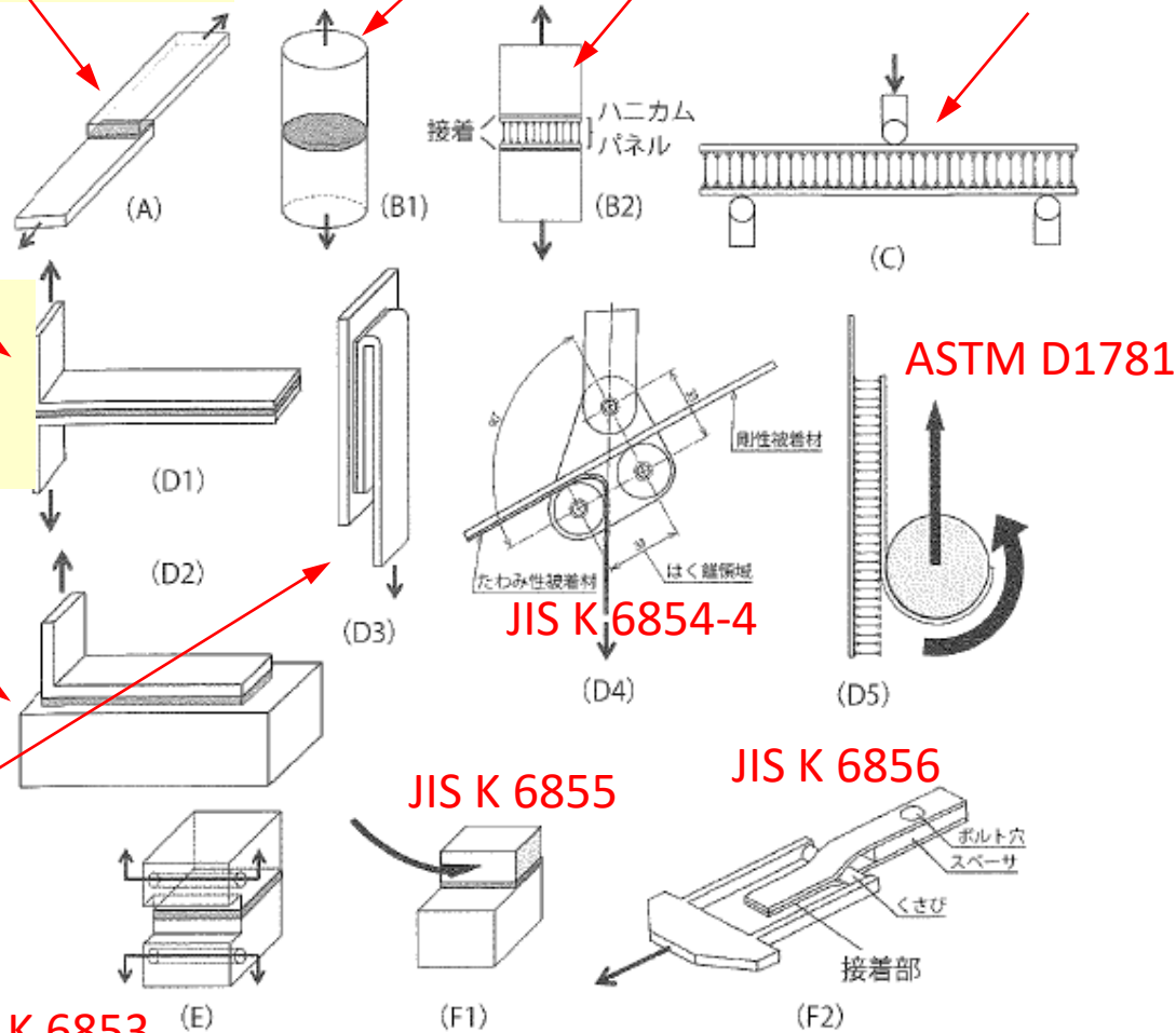
図 2.3.1 接着強度の各種測定方法
